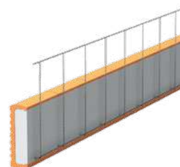
Porotherm KP Vario 200-350 (rozмеры v reze: 70 x 238 mm)
